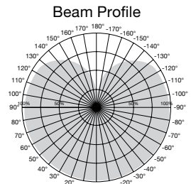
Beam Angle: 280°
