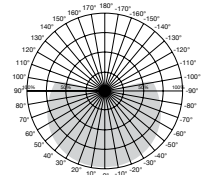
Beam Angle: 107°
